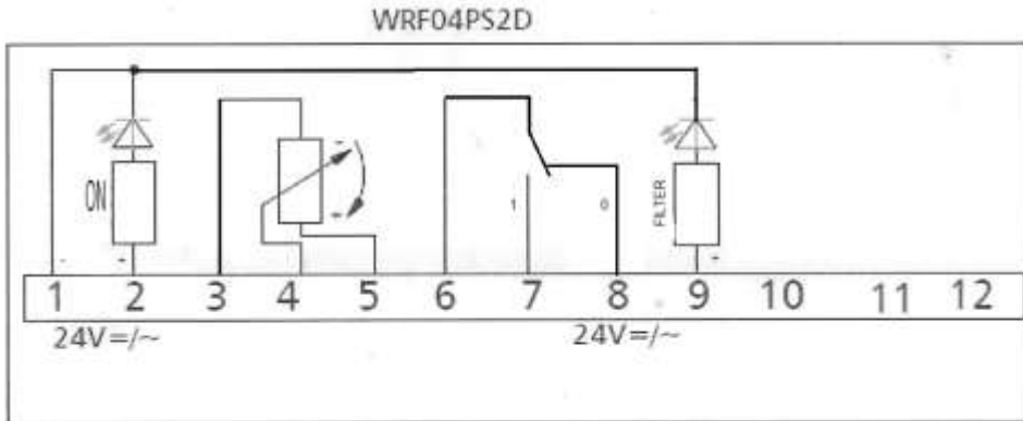
Afb. 11 Wandbediening aansluitschema, aangegeven in de wandbediening.
